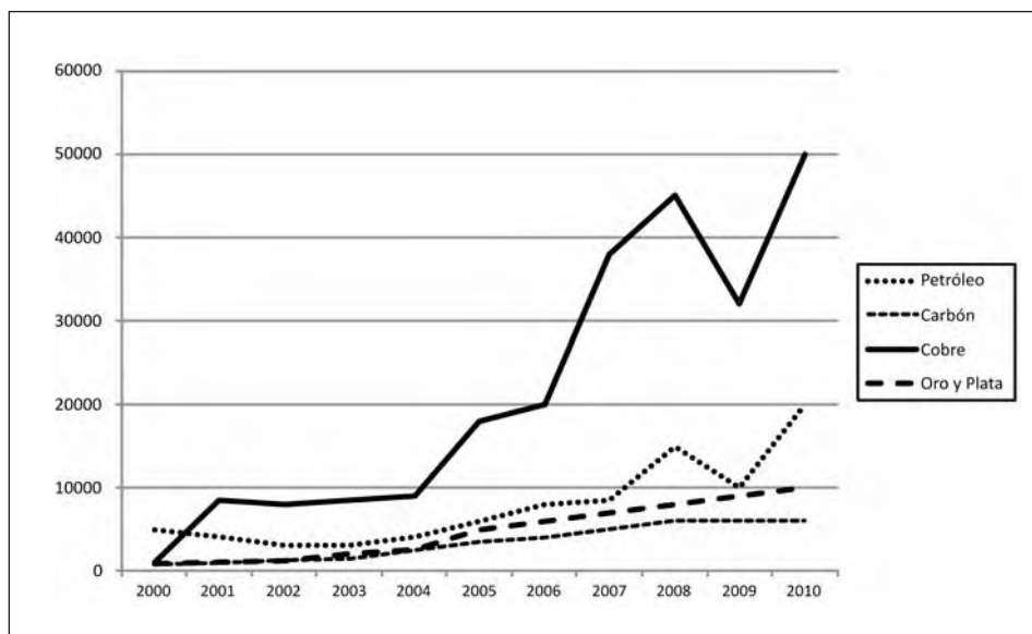
Gráfica 3 Exportaciones mineras Colombia, Perú y Chile 2000-2011
